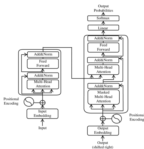
Figura 1. Estrutura Transformer
